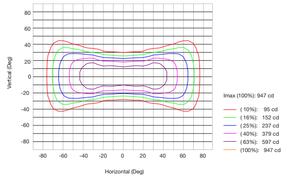
FLARE Flare Optics 100° x 20° Beam Angle
